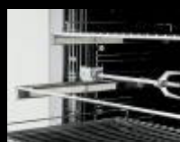
Gradins télescopiques : encore plus de sécurité grâce à une meilleure stabilité des grilles et du tournebroche.
